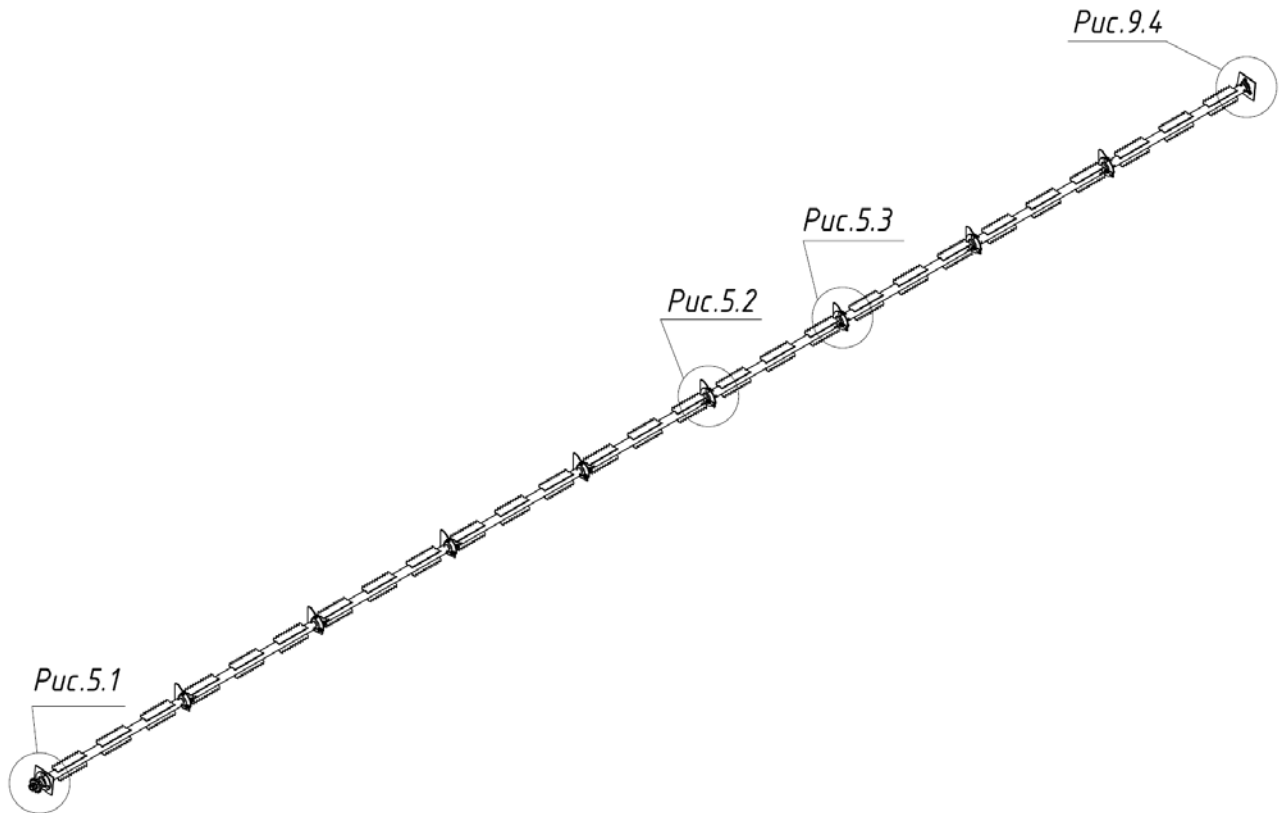
Рис.5 Вал протягивающий.
