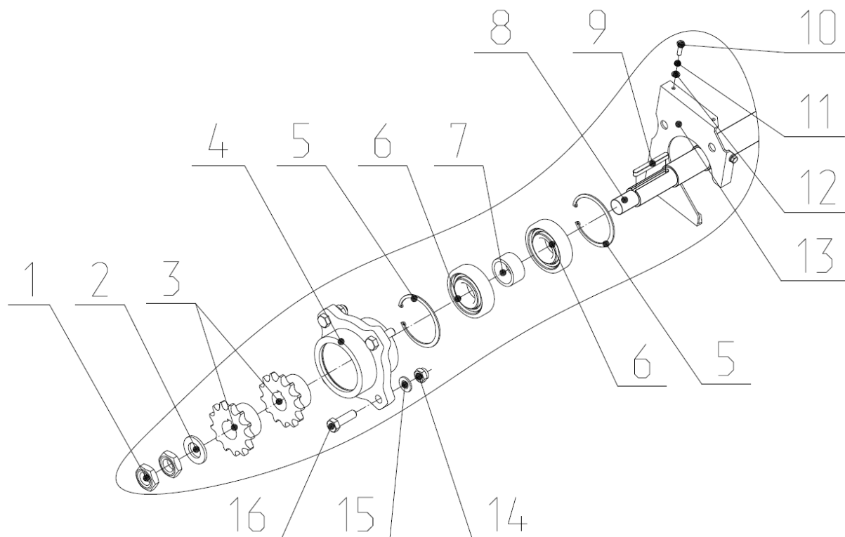
Рис.3а ЖНПС 00.010 Вал в сборе.
