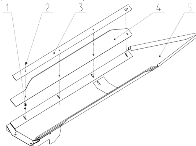
Рис.3.1 Поддон в сборе.
