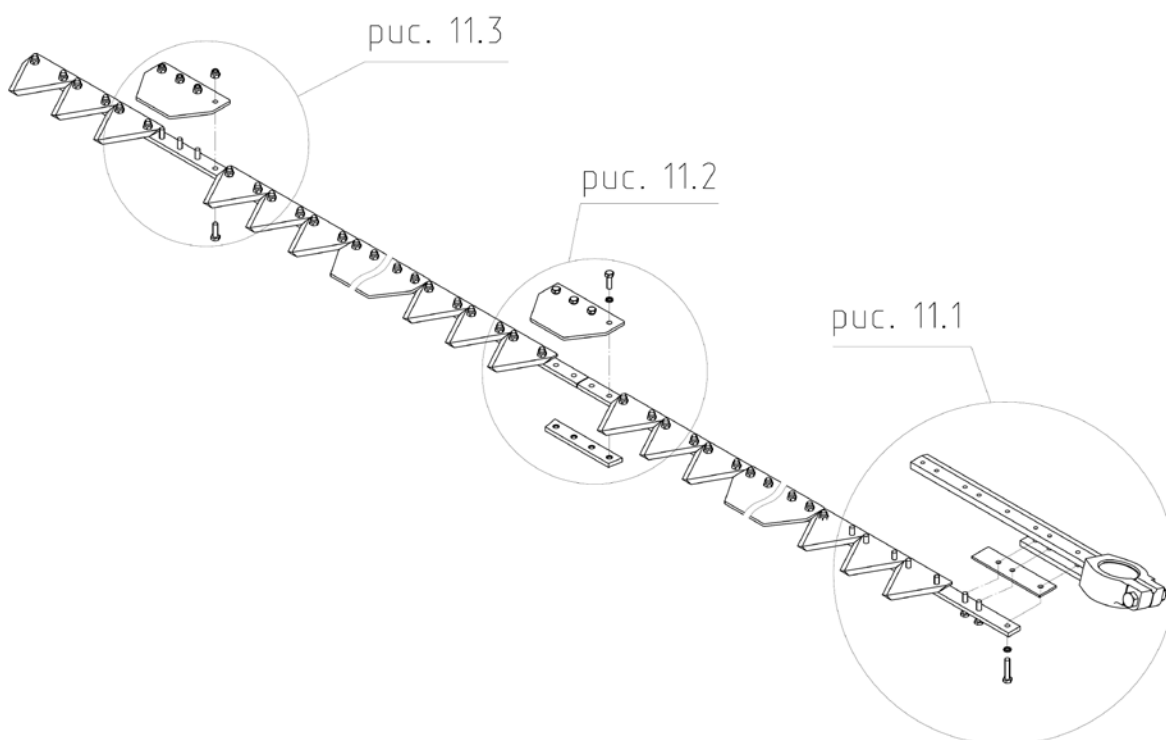
Рис. 2.1 ЖНС 06.010 Режущий аппарат.
