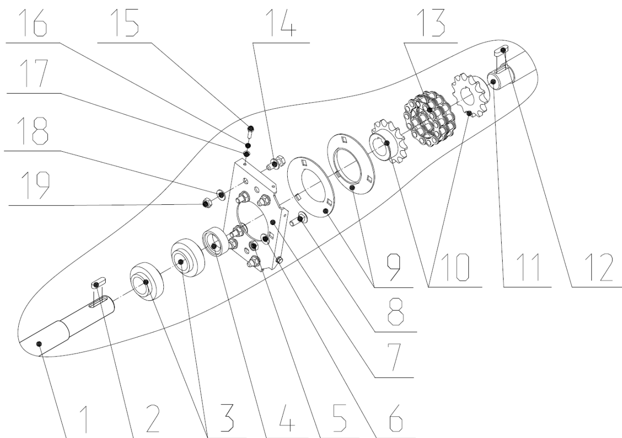
Рис.3.6 ЖНПС 00.020 Вал в сборе.
