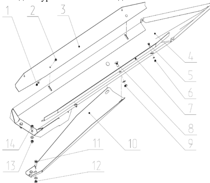
Рис.3 ЖНПС 02.010 Поддон в сборе.
