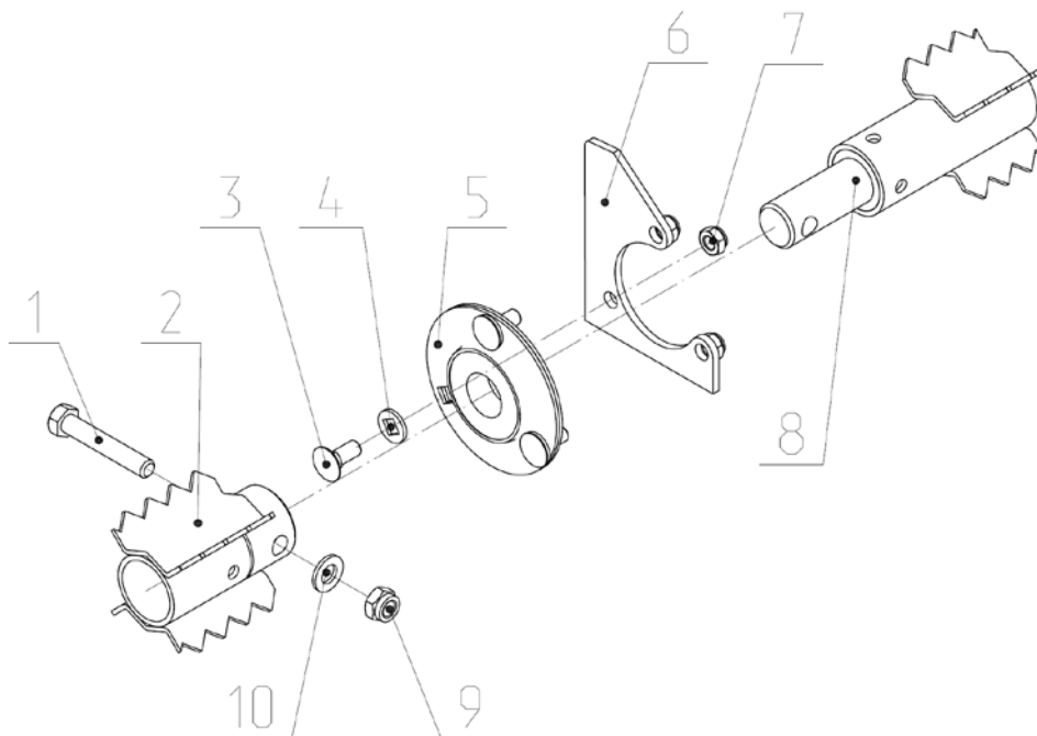
Рис. 5.3 Вал протягивающий соединение втулка-вал.
