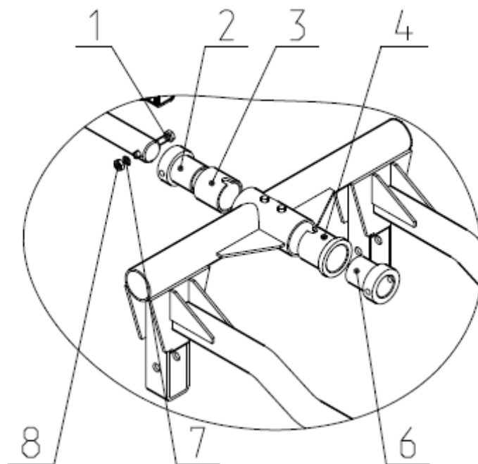
Рис.19б Держатель.
