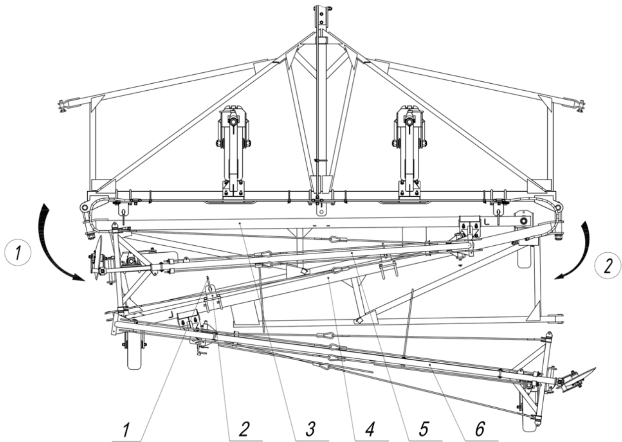
Рис. 13а Схема перевода сцепки в транспортное положение.
