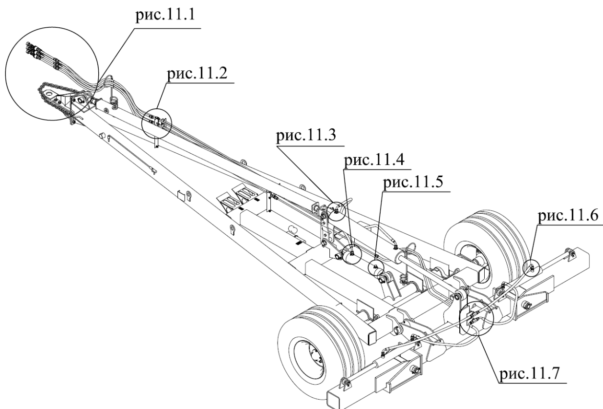
Рис.11 Гидросистема.
