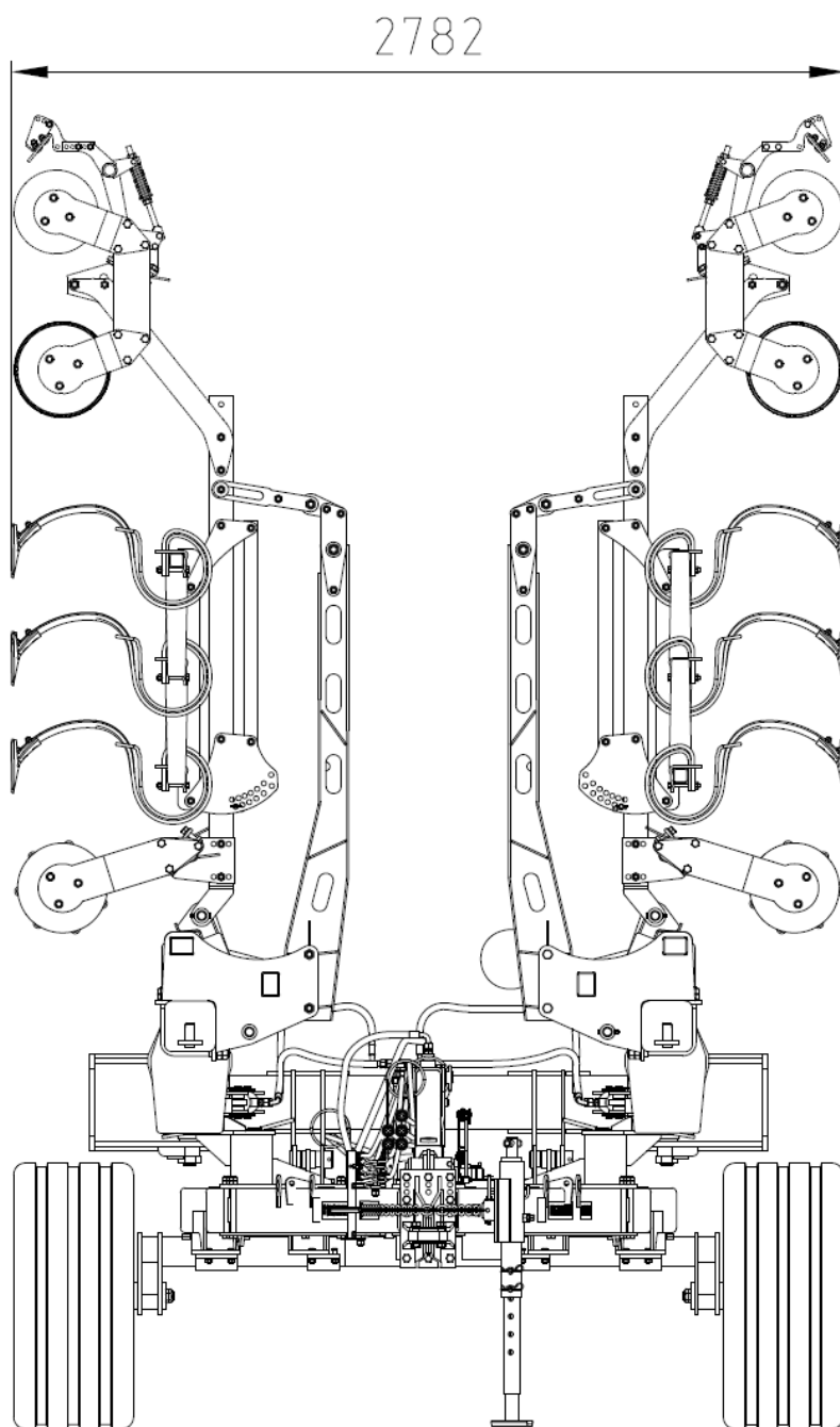
КБП8 с демонстрированными катками. Вид спереди.
