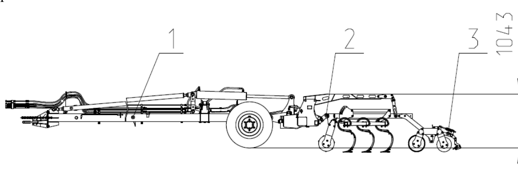
Рис.2 Культиватор КБП8-4 К1 (Вид сбоку)
