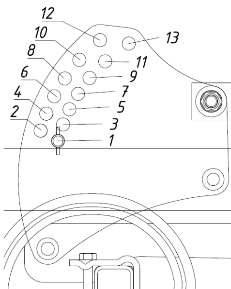
Рис.15.2 Соответствие отверстий глубине обработки
