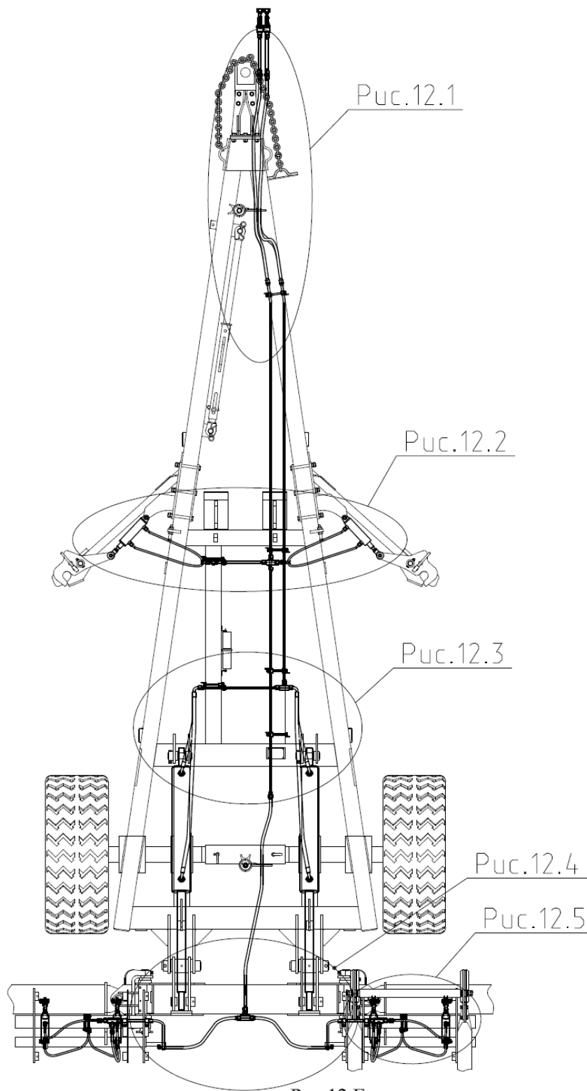
Рис.12 Гидросистема.
