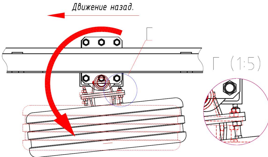
Рис.16 Регулировка транспортных колес боковых балок
