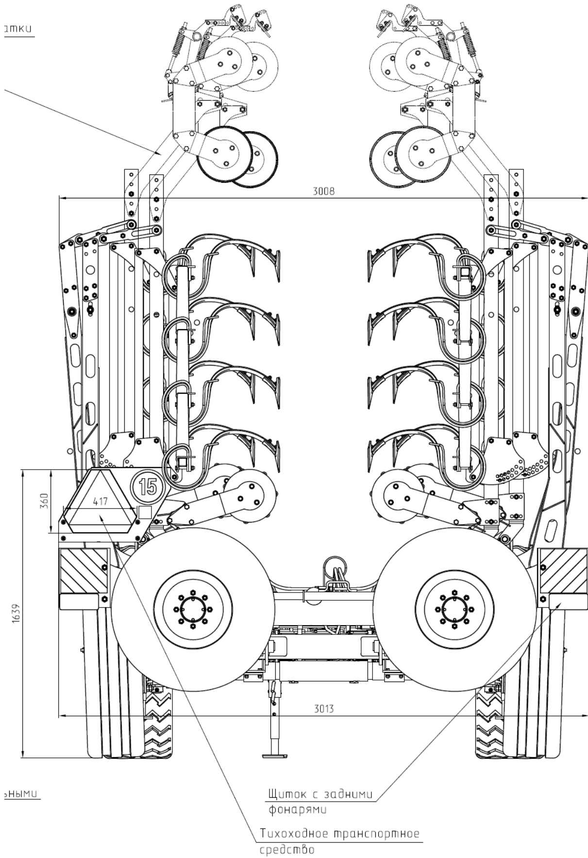
КБП12 с демонтированными катками. Вид сзади
