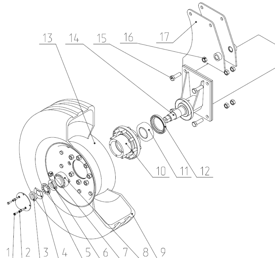
Рис.8 Колесо в сборе СГВ 03.010
