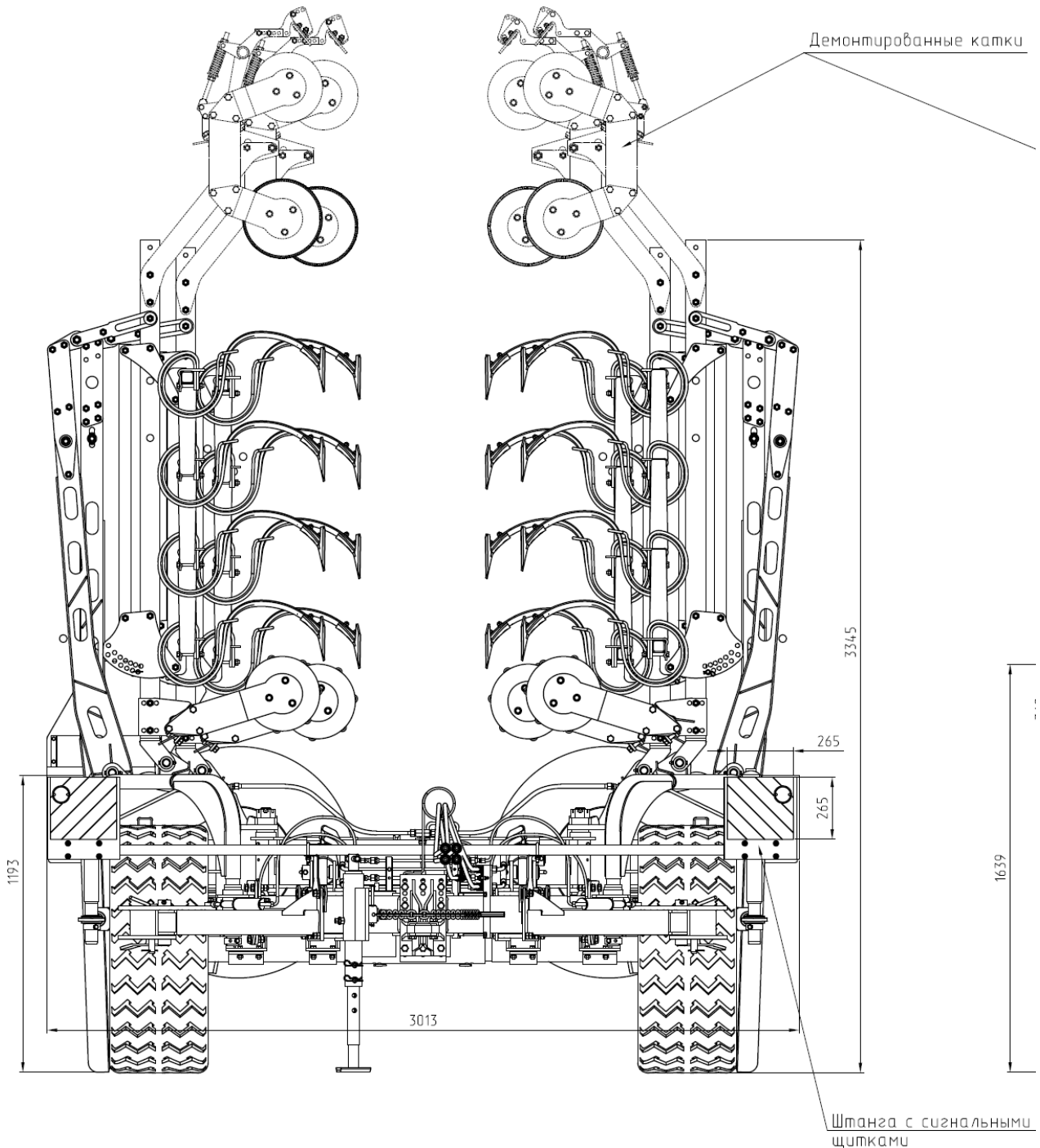
КБП12 с демонтированными катками. Вид спереди
