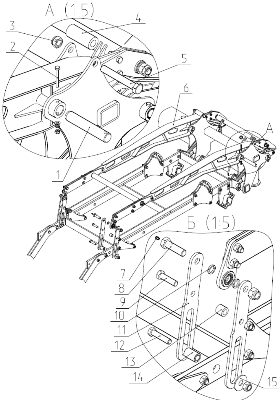
Рис.11.8 Установка подвески КБП 02.160-01.
