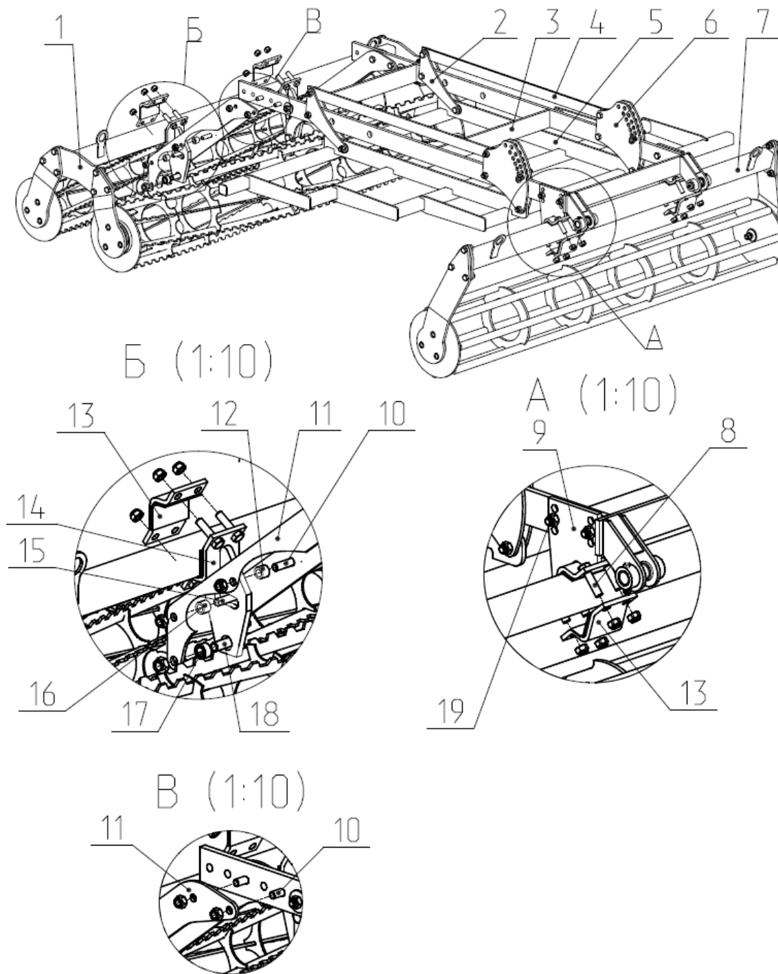
Рис.11.1 Установка катков.
