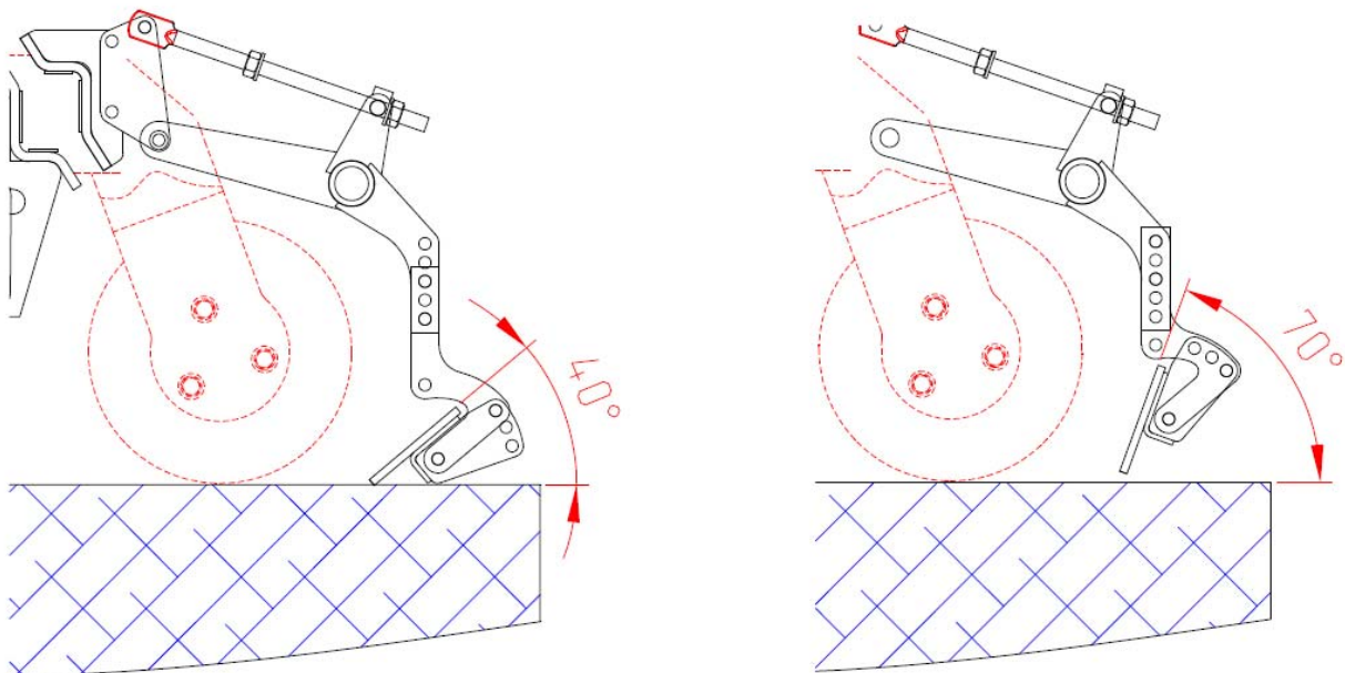
Рис.24а Регулировка планчатого выравнителя по углу (активное положение планки).
