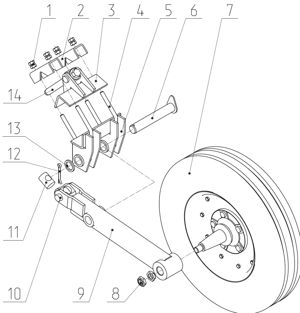
Рис.9 Колесо опорное боковых секций.
