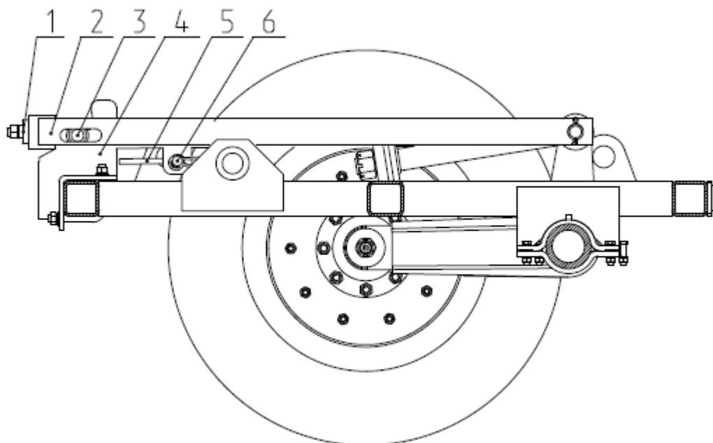
Рис.7 Положение транспортного фиксатора при работе культиватора.
