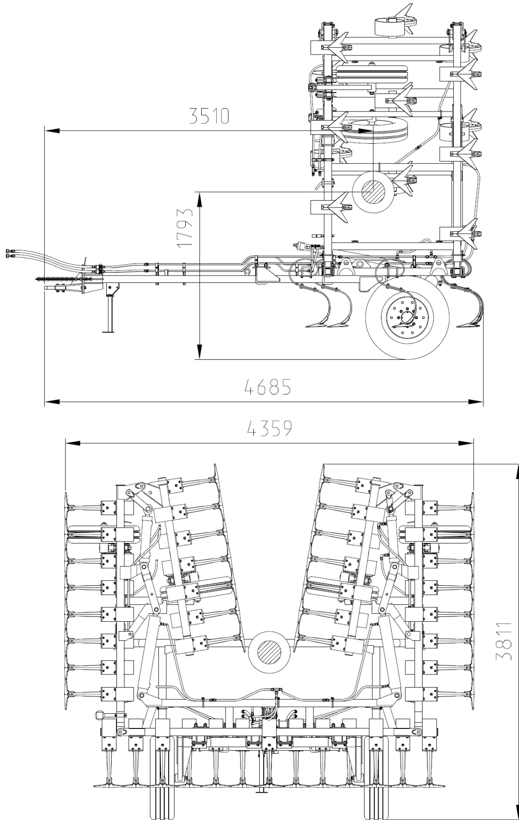
Рис1-1а Расположение центр масс КСП-12-01.
