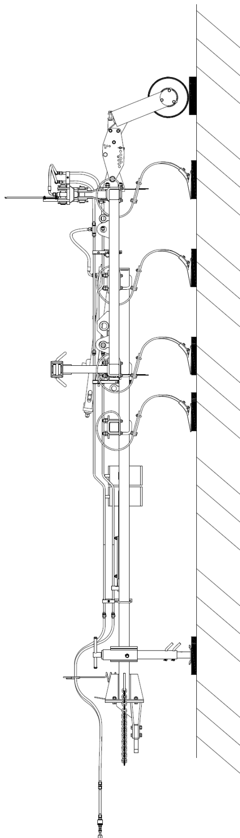
Рис.26 Установка культиватора на хранение.
