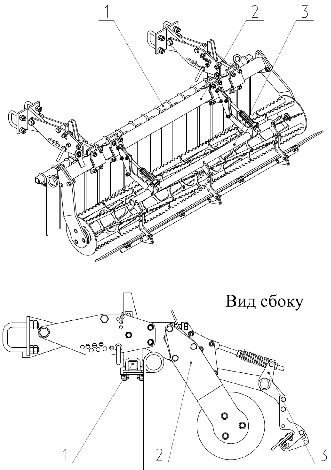
Рис.15 Установка секций однорядной гребенки к однорядному катку и к планчатому выравнителю.
