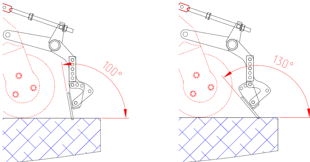
Рис.246 Регулировка планчатого выравнителя по углу (пассивное положение планки).
