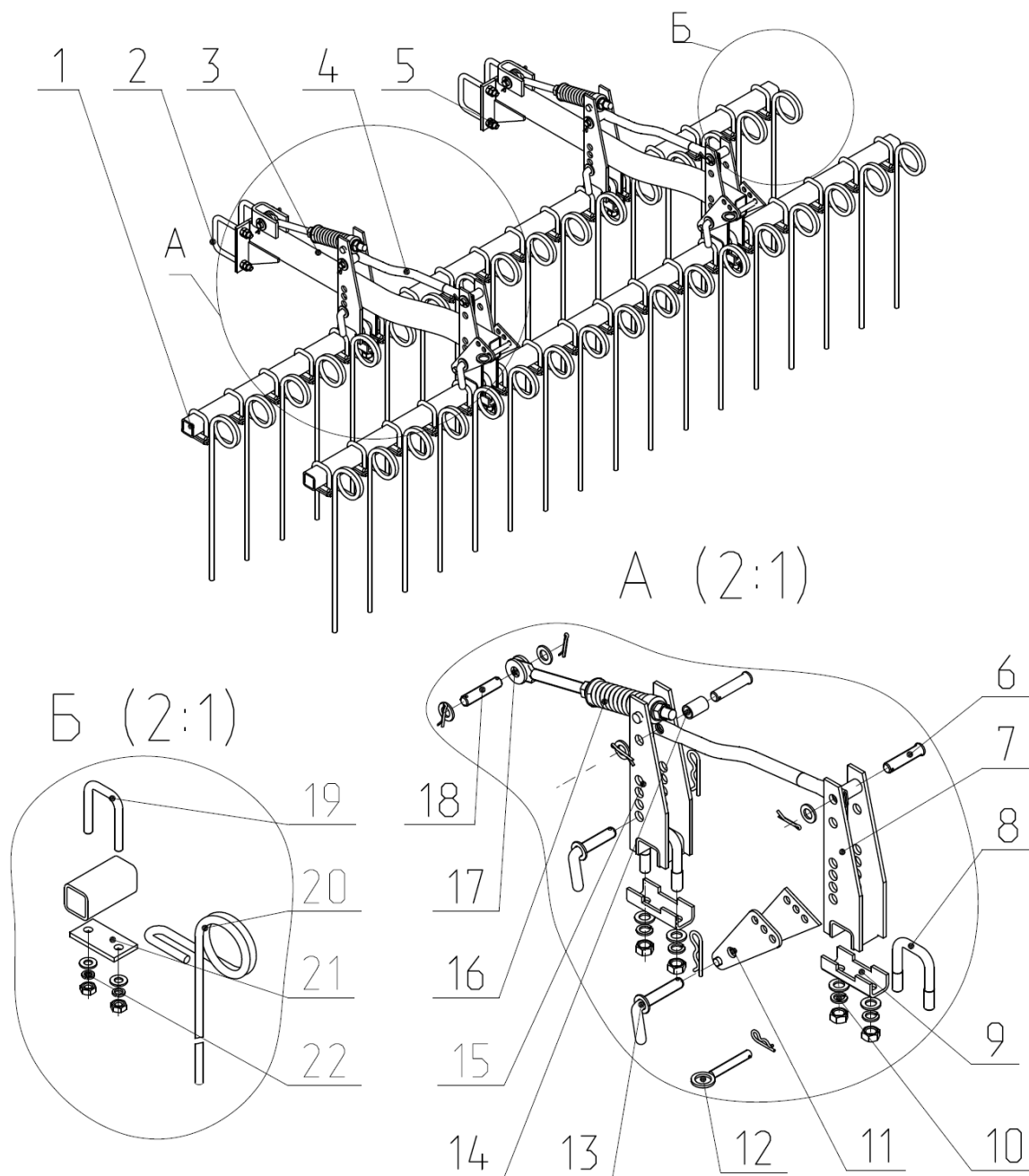
Рис.16 КСП 08.010 Двухрядная гребенка.
