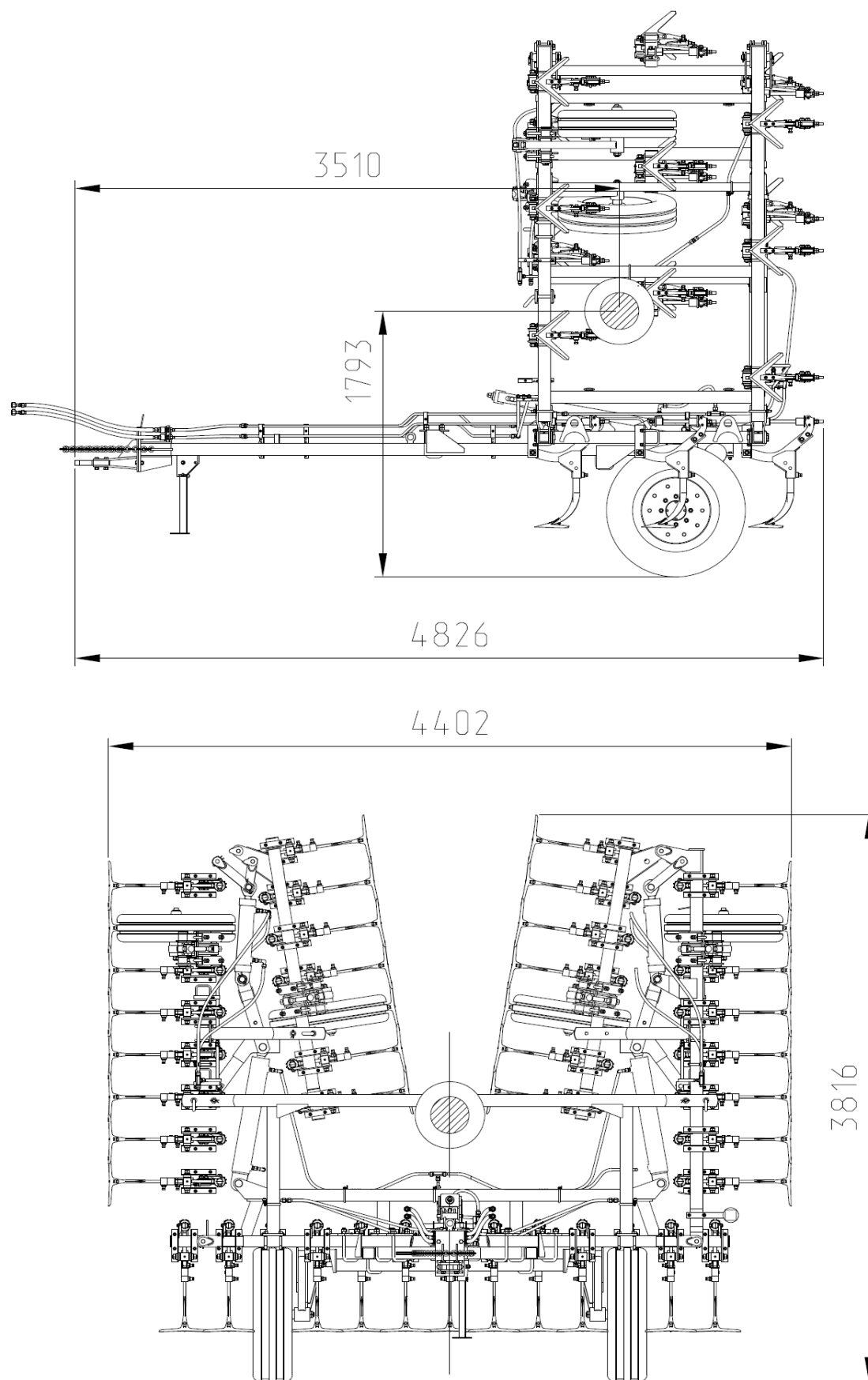
Рис.1а Расположение центр масс КСП-12.
