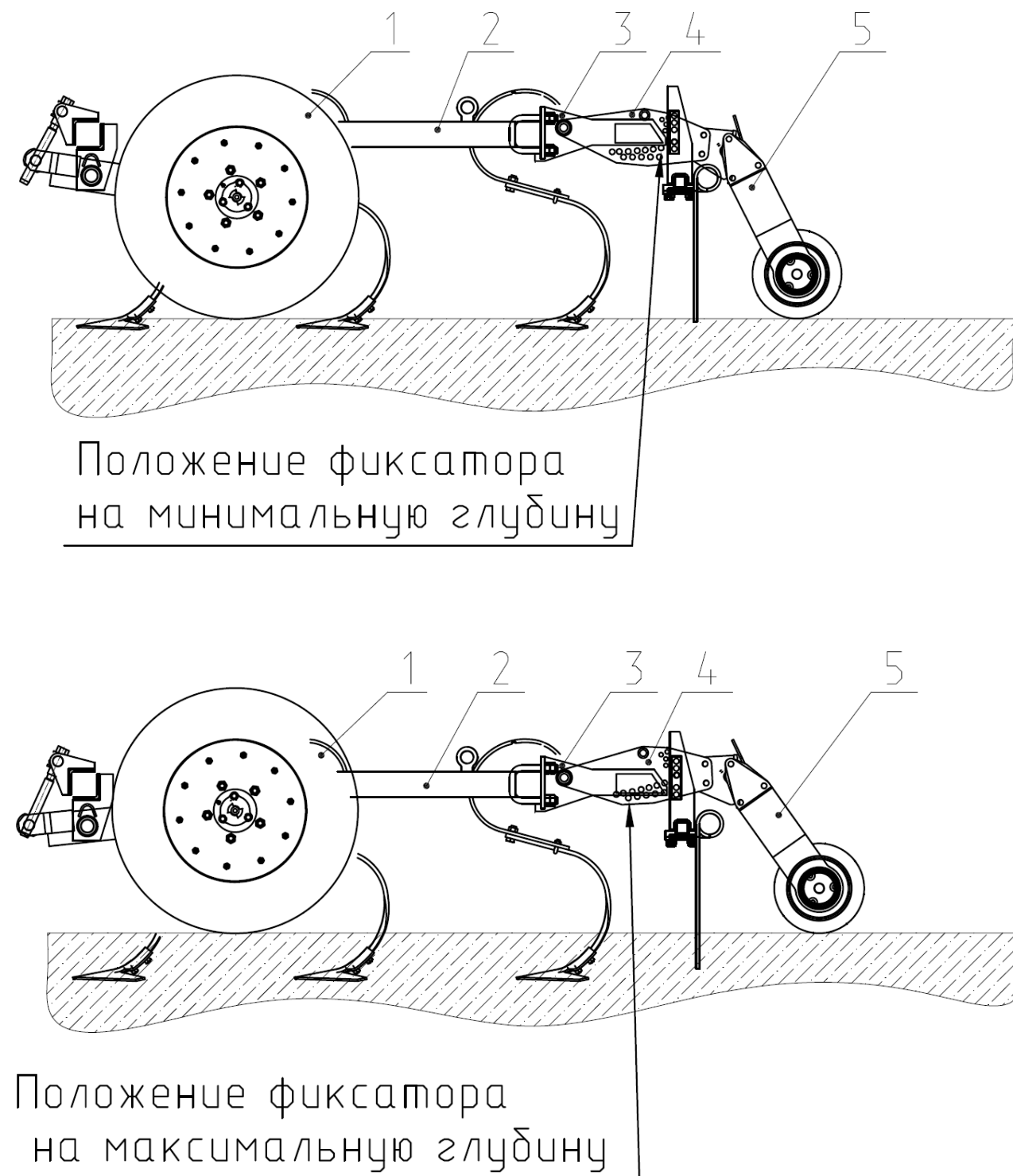
Рис.22 Установка глубины обработки рабочих органов катками однорядными.
