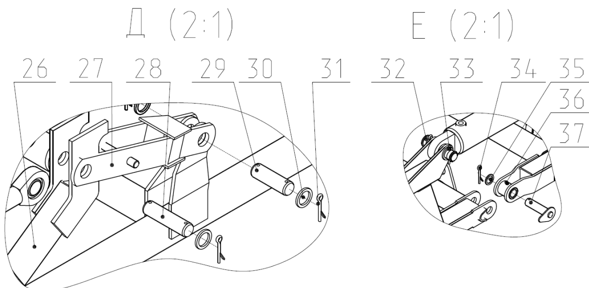
Рис.3а Центральная и боковые секции (продолжение).
