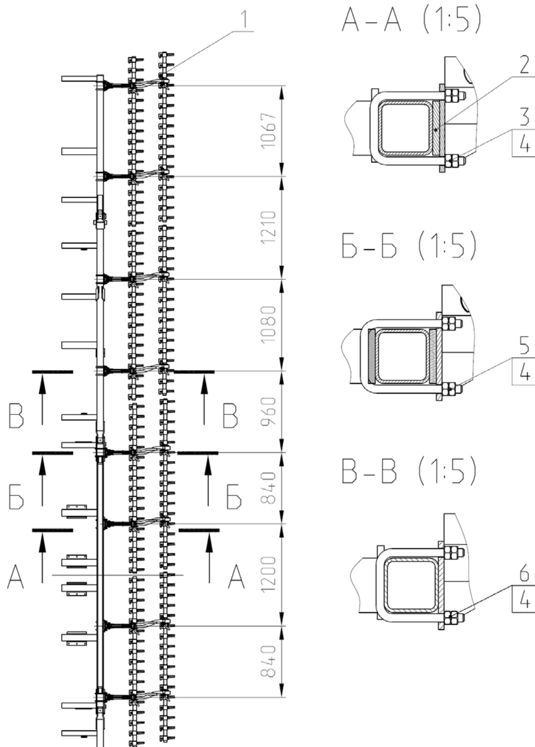
Рис.19 Установка двухрядной гребенки КСП 08.010.
