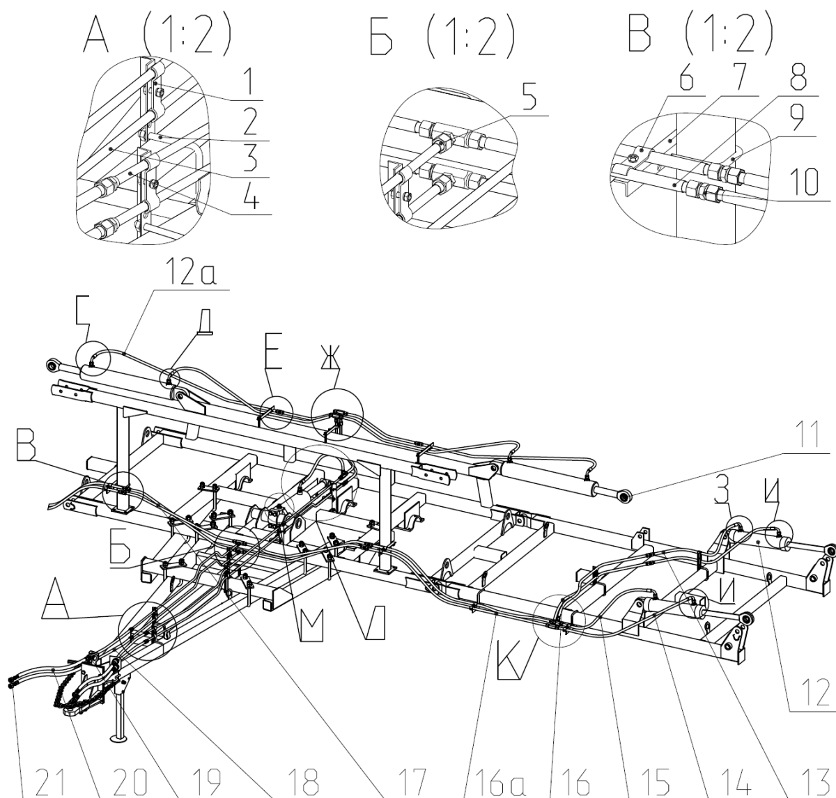
Рис.20 Гидросистема КСП-12
