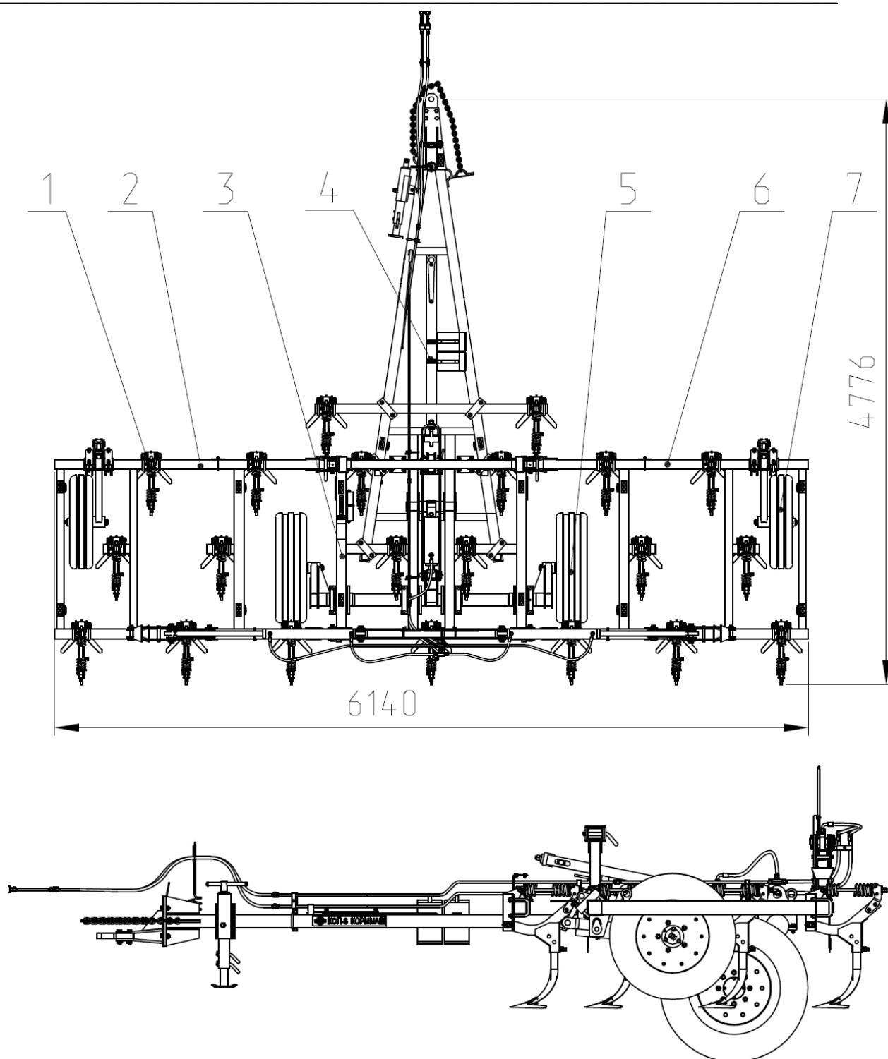
Рис.1а Культиватор КСП-6
