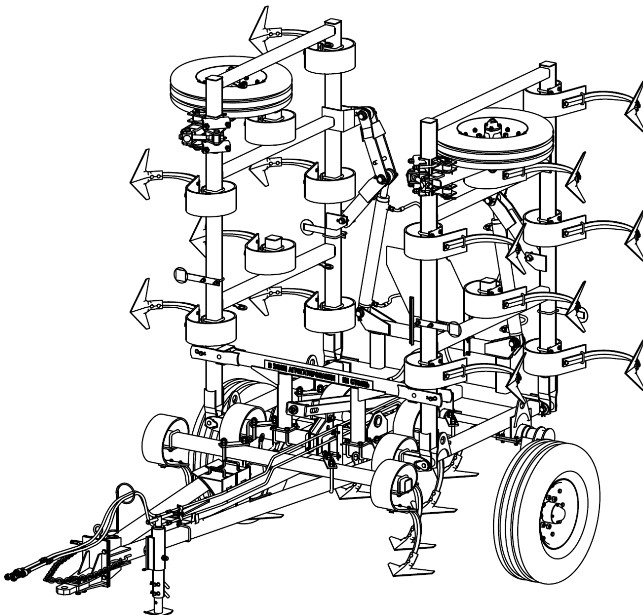
Рис.26 Культиватор для сплошной обработки почвы КСП-6-01 "Чеглок" (в транспортном положении).
