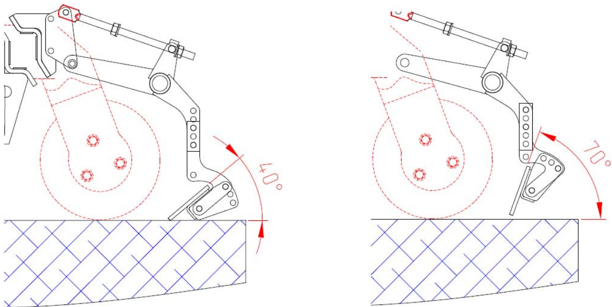
Рис.28а Регулировка планчатого выравнивателя по углу (активное положение планки).
