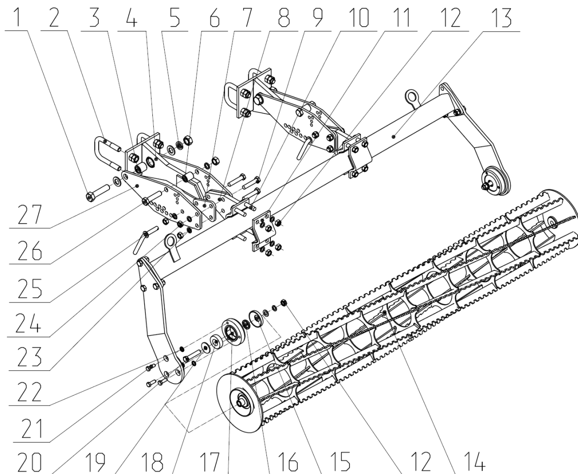
Рис.12 КСП 04.160 Секция катка однорядного.
