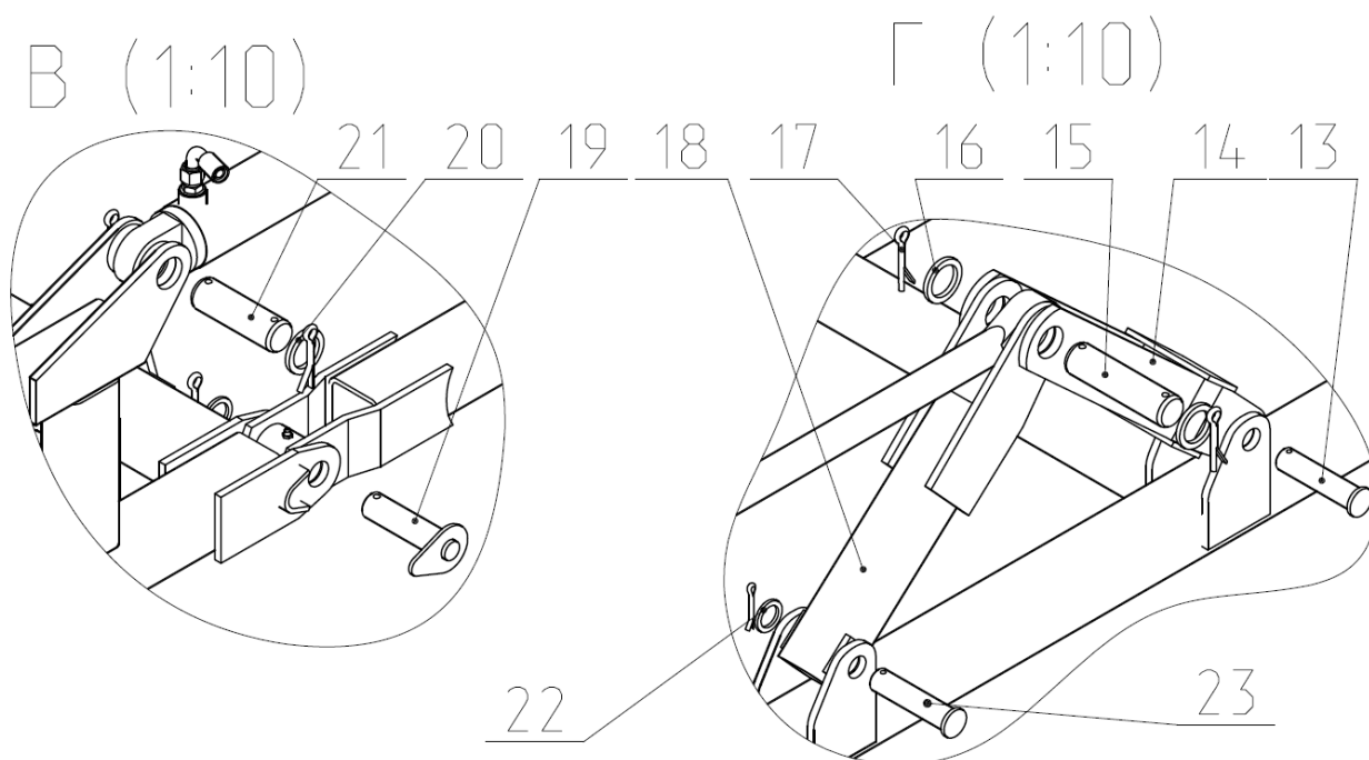
Рис.3 Сборка центральной секции с крылом (продолжение).
