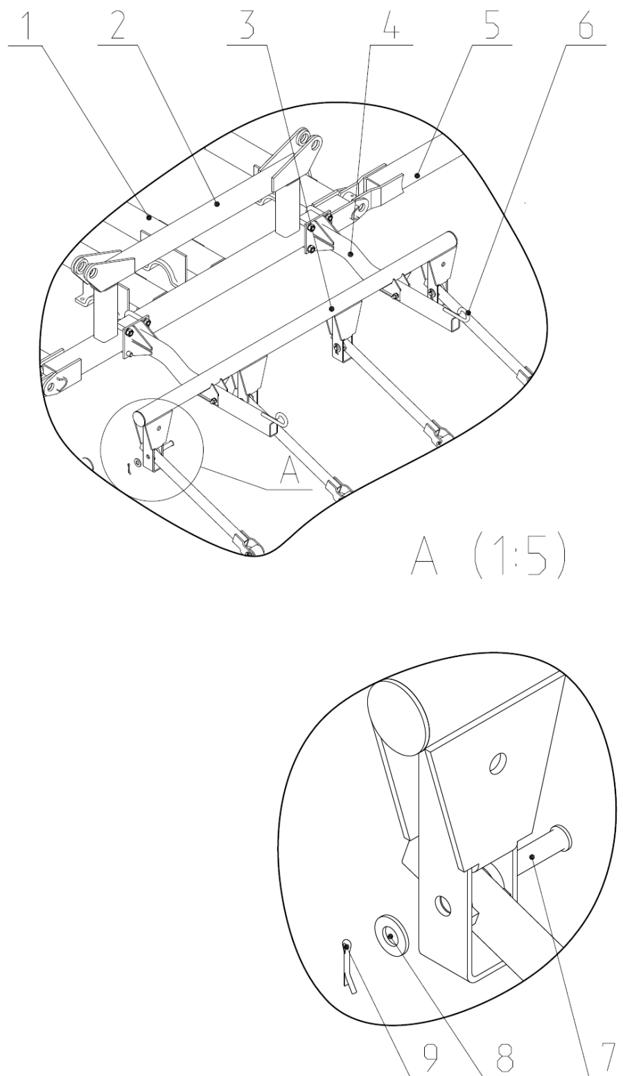
Рис.19в Навеска зубовых борон.
