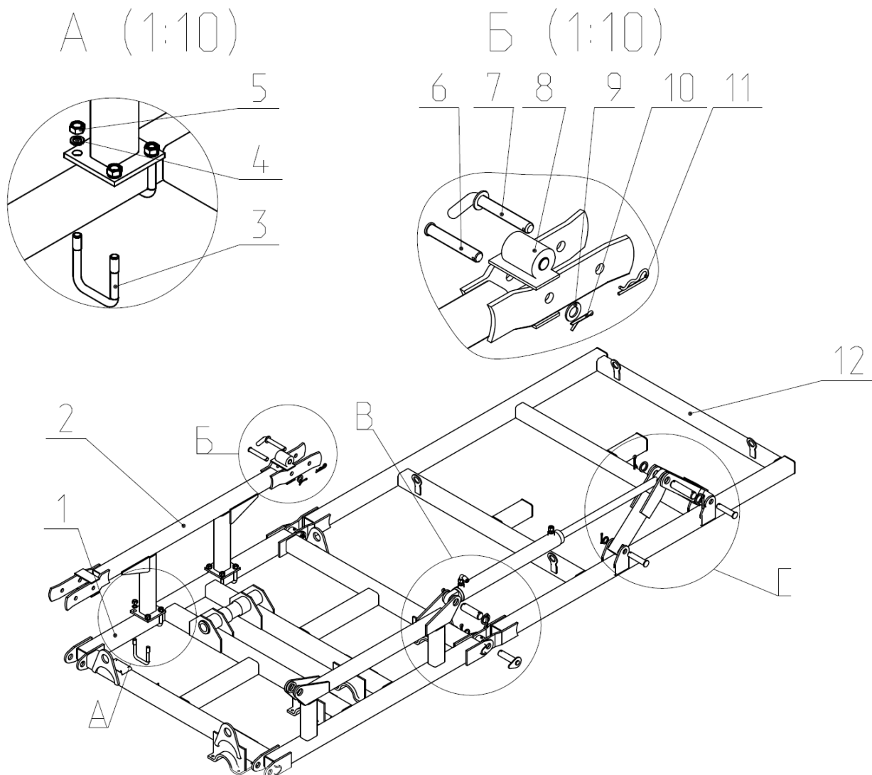
Рис.3 Сборка центральной секции с крылом.
