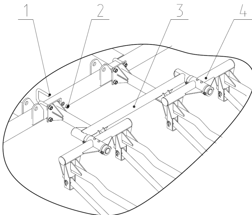
Рис. 19а Установка на крыльях.
