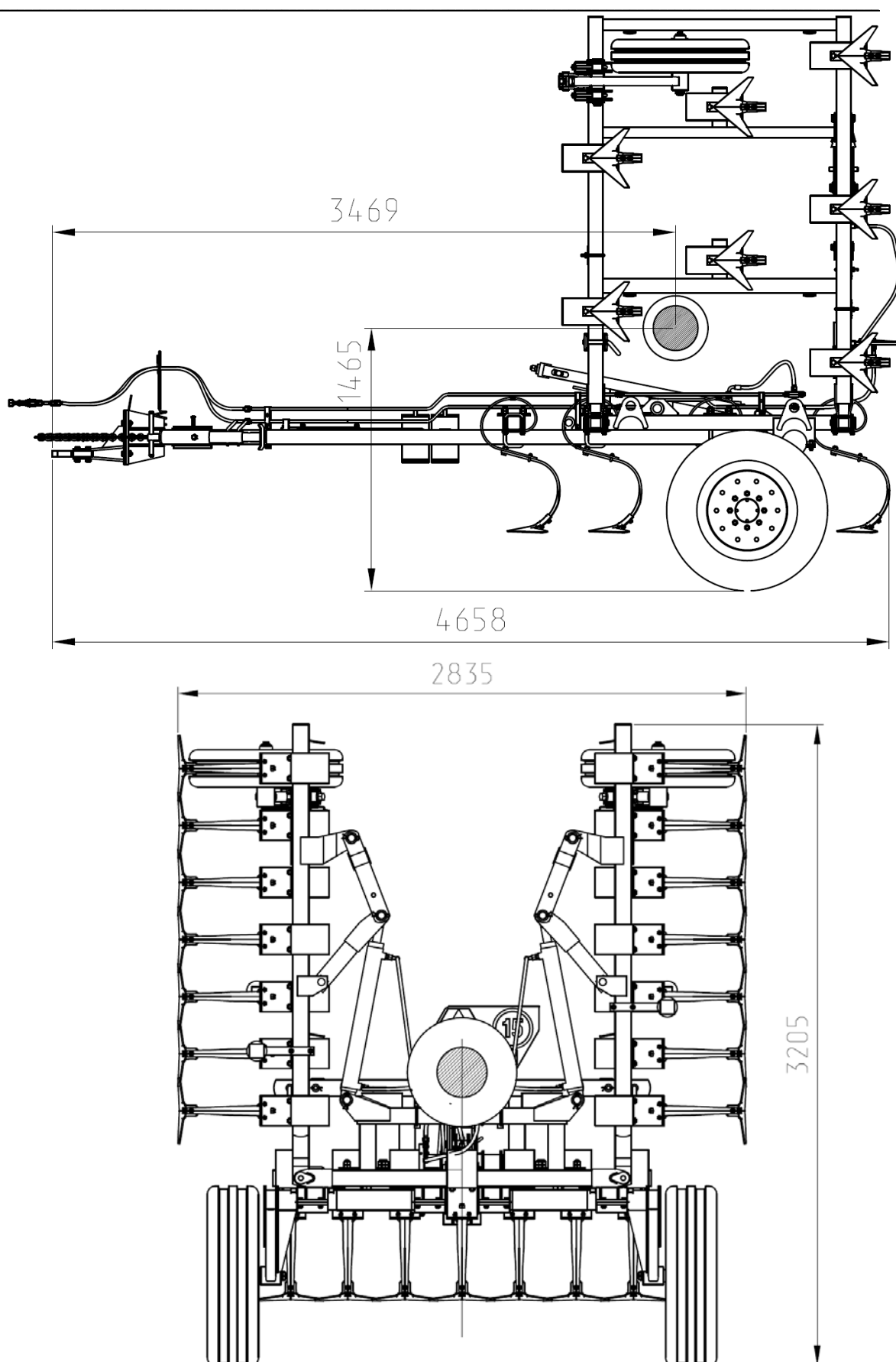
Рис.2 КСП-6-01 Расположение центр масс.
