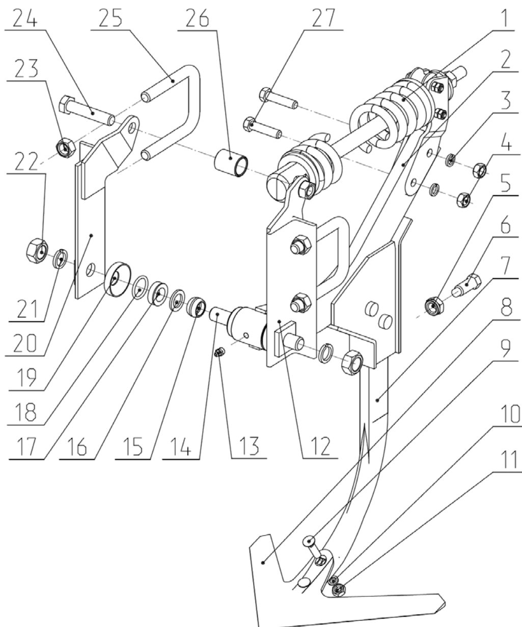
Рис.11 КСП 00.010А Рабочий орган.
