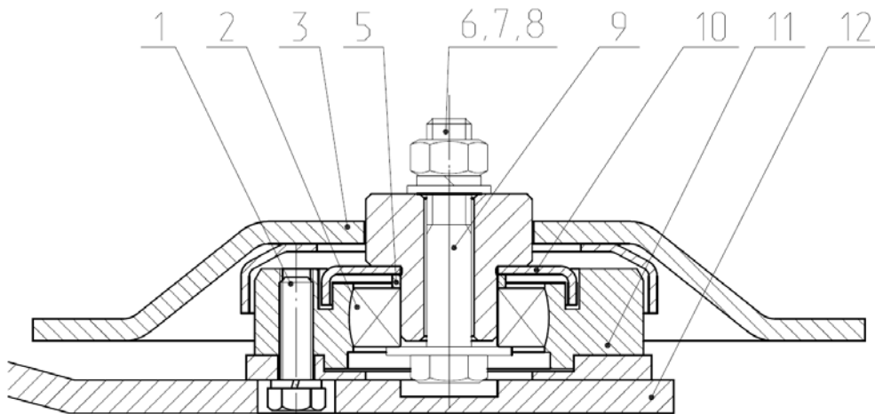
Рис.13в Подшипниковый узел.
