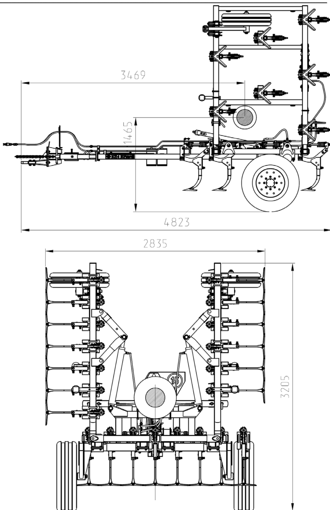
Рис.2а КСП-6 Расположение центр масс.
