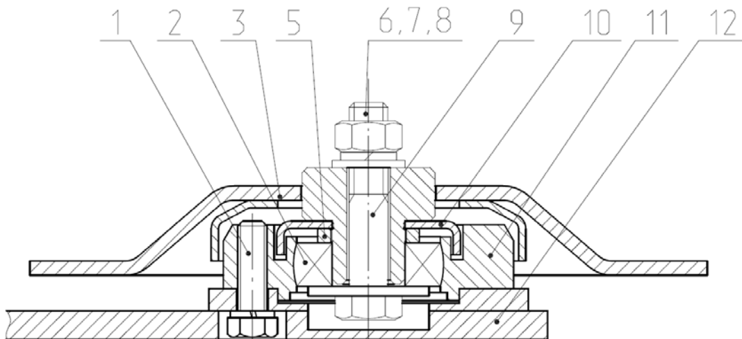
Рис.13г Подшипниковый узел.
