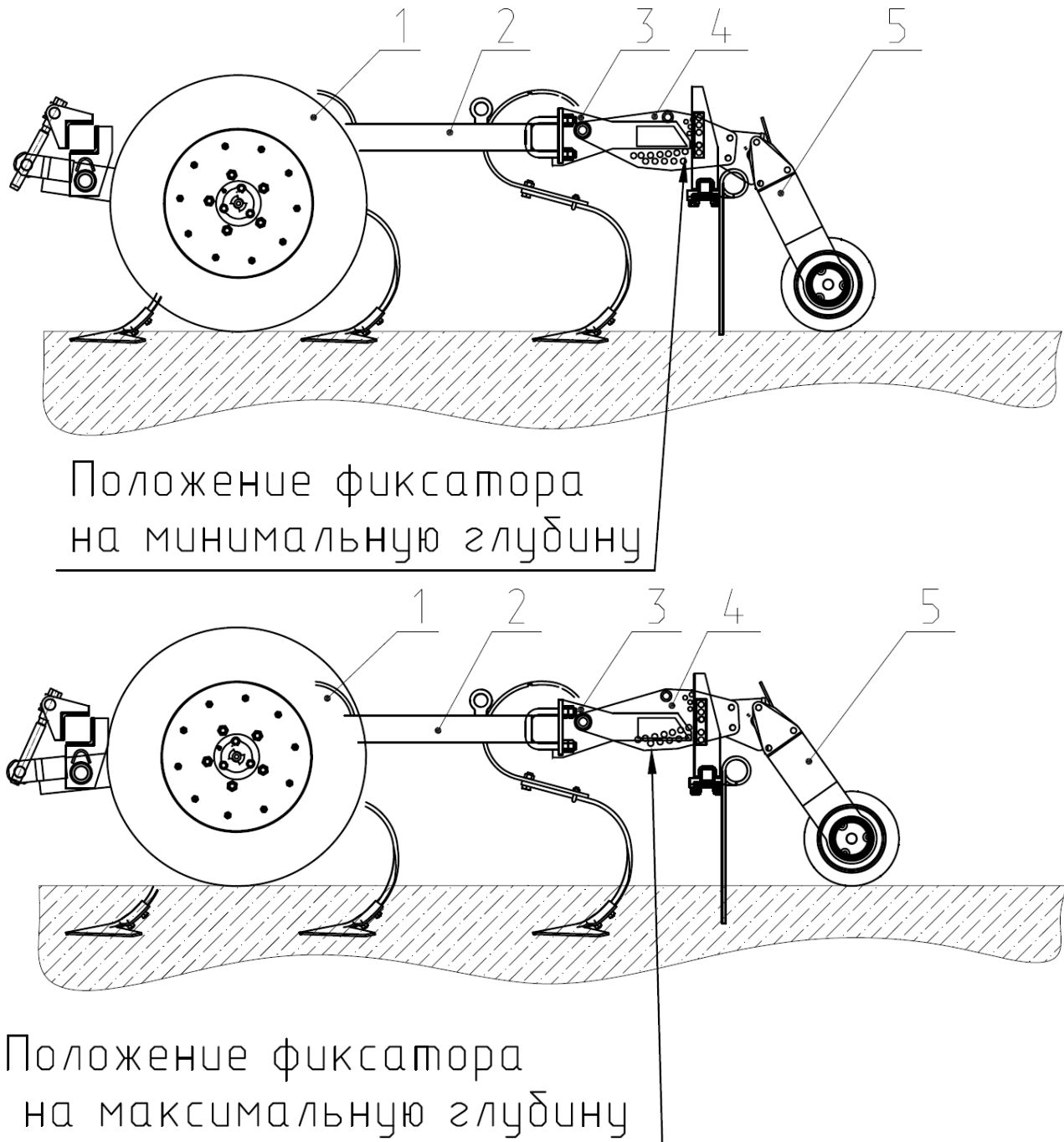
Рис.25 Установка глубины обработки рабочих органов катками однорядными.
