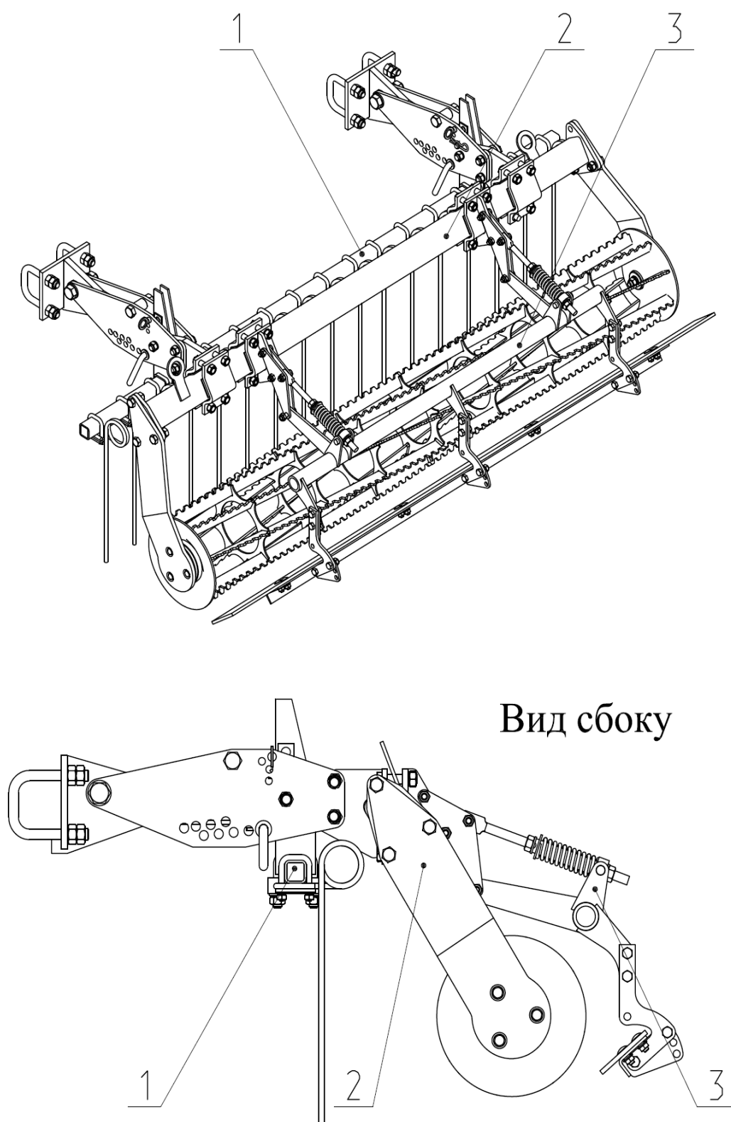
Рис.16 Секция катков однорядных в комплекте с однорядной гребенкой и планчатым выравнивателем.
