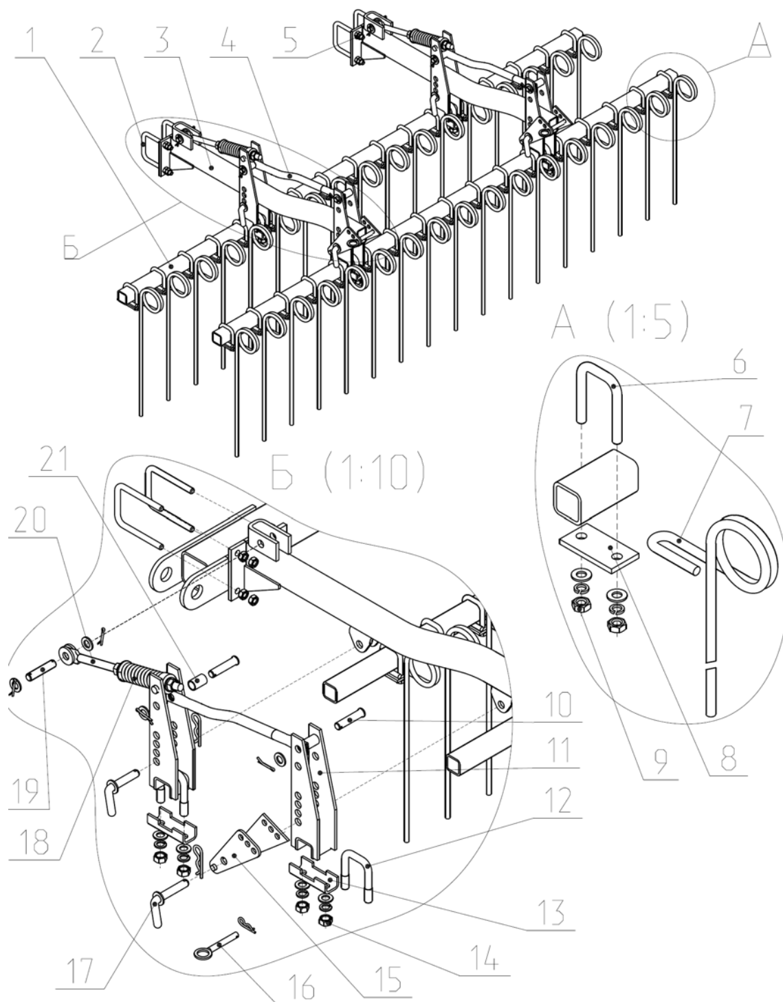
Рис.18 КСП 08.010 Гребенка двухрядная.
