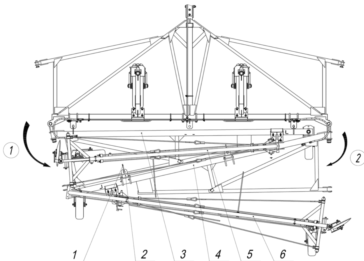
Рис. 13а Схема перевода сцепки в транспортное положение.
