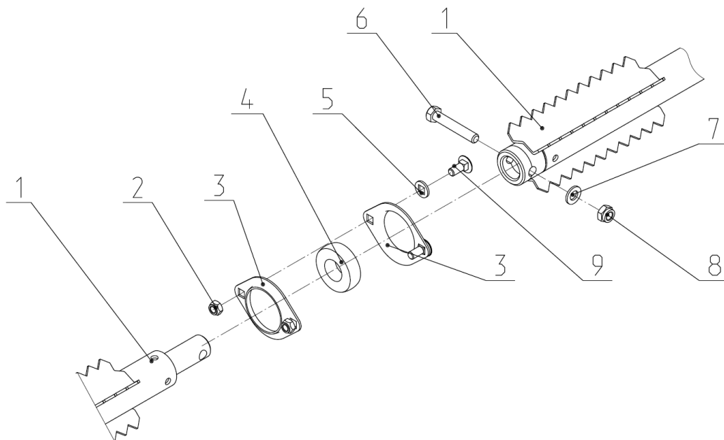
Рис. 5.2 Вал протягивающий соединение.
