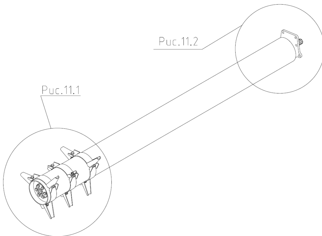
Рис.11 ЖНП 03.020А-02 Мотовило.
