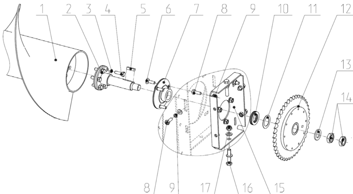
Рис.13.3 ЖНС 04.000 Шнек в сборе.
