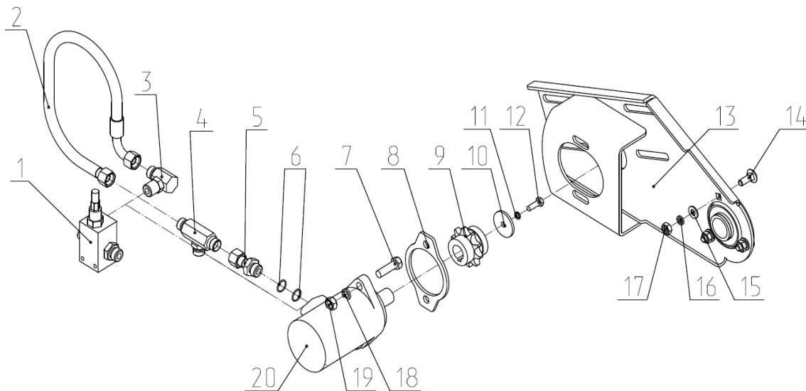
Рис.9 ЖНС 00.390 Гидромотор.
