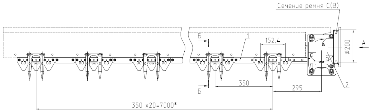
Рис. 2 ЖНС 06.000 Режущий аппарат в сборе.
