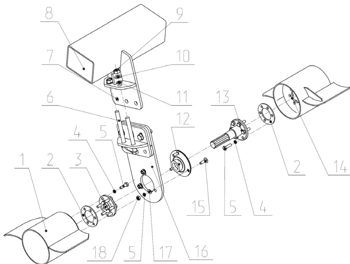
Рис.13.2 ЖНС 04.000 Шнек в сборе.
