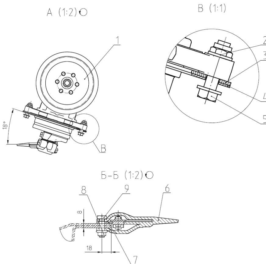
Рис.2.1 ЖНС 06.000 Режущий аппарат в сборе
