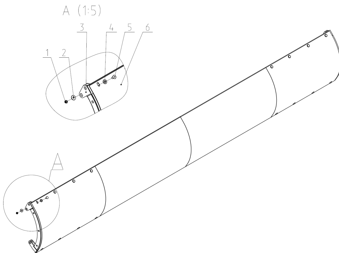
Рис. 7 ЖНС 03.190 Щиток
