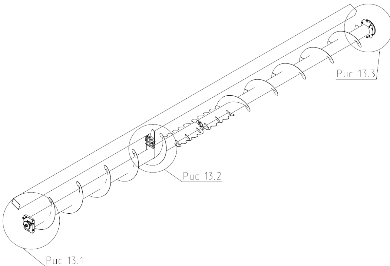
Рис.13 ЖНС 04.000 Шнек в сборе.
