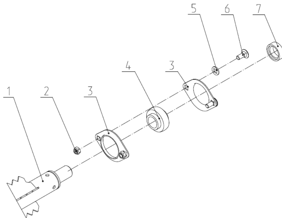
Рис.5.3 Вал протягивающий.
