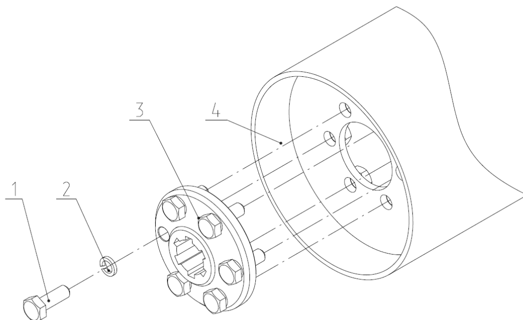
Рис.12.1 ЖНС 03.020-02 Мотовило.
