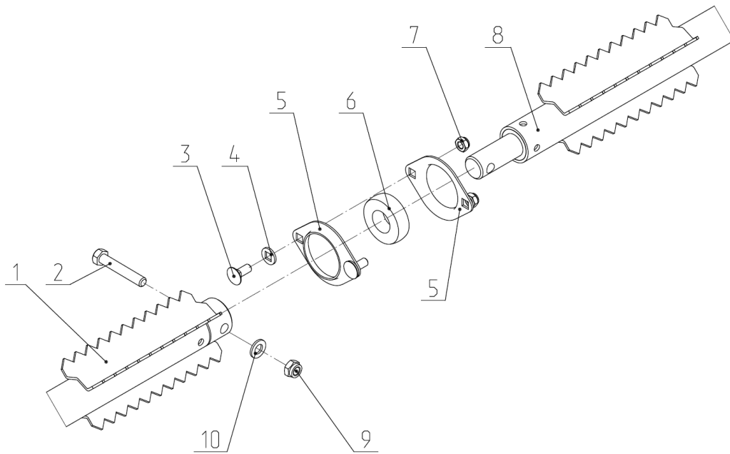
Рис. 5.3 Вал протягивающий соединение.
