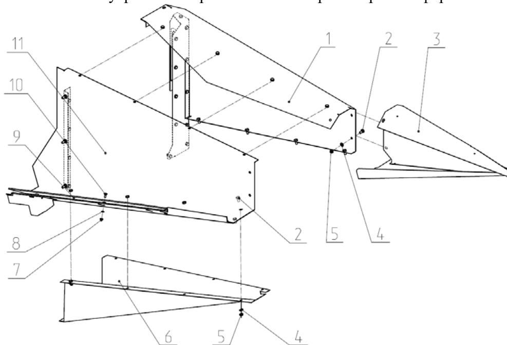
Рис. 4 ЖНПС 02.070 Пиллета.
