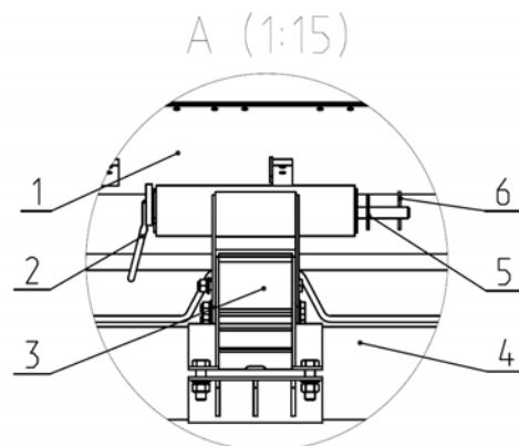
(См. РЭ ТТ-3000 Рис.18 Установка жатки на приспособление.)
