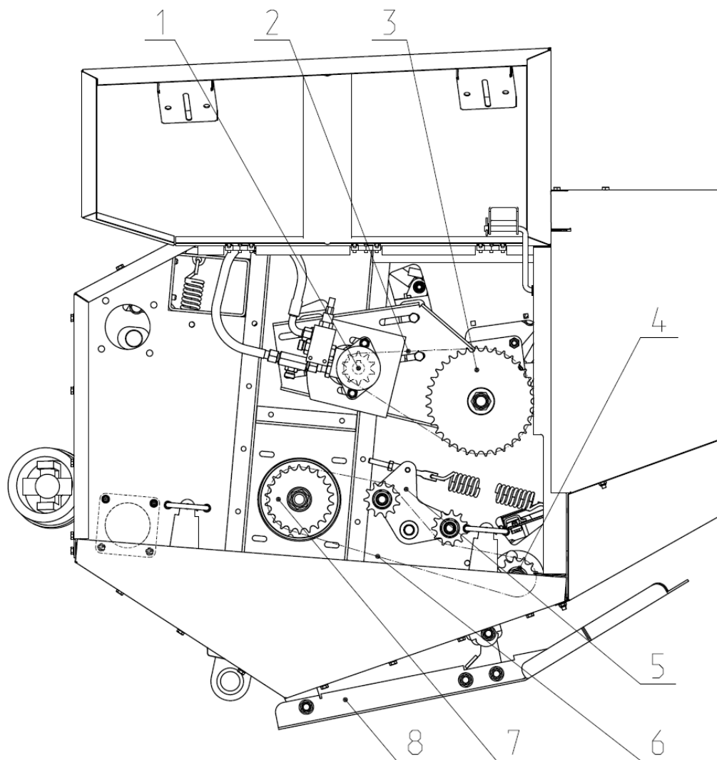
Рис. 1.4 Привод правой части жатки.
