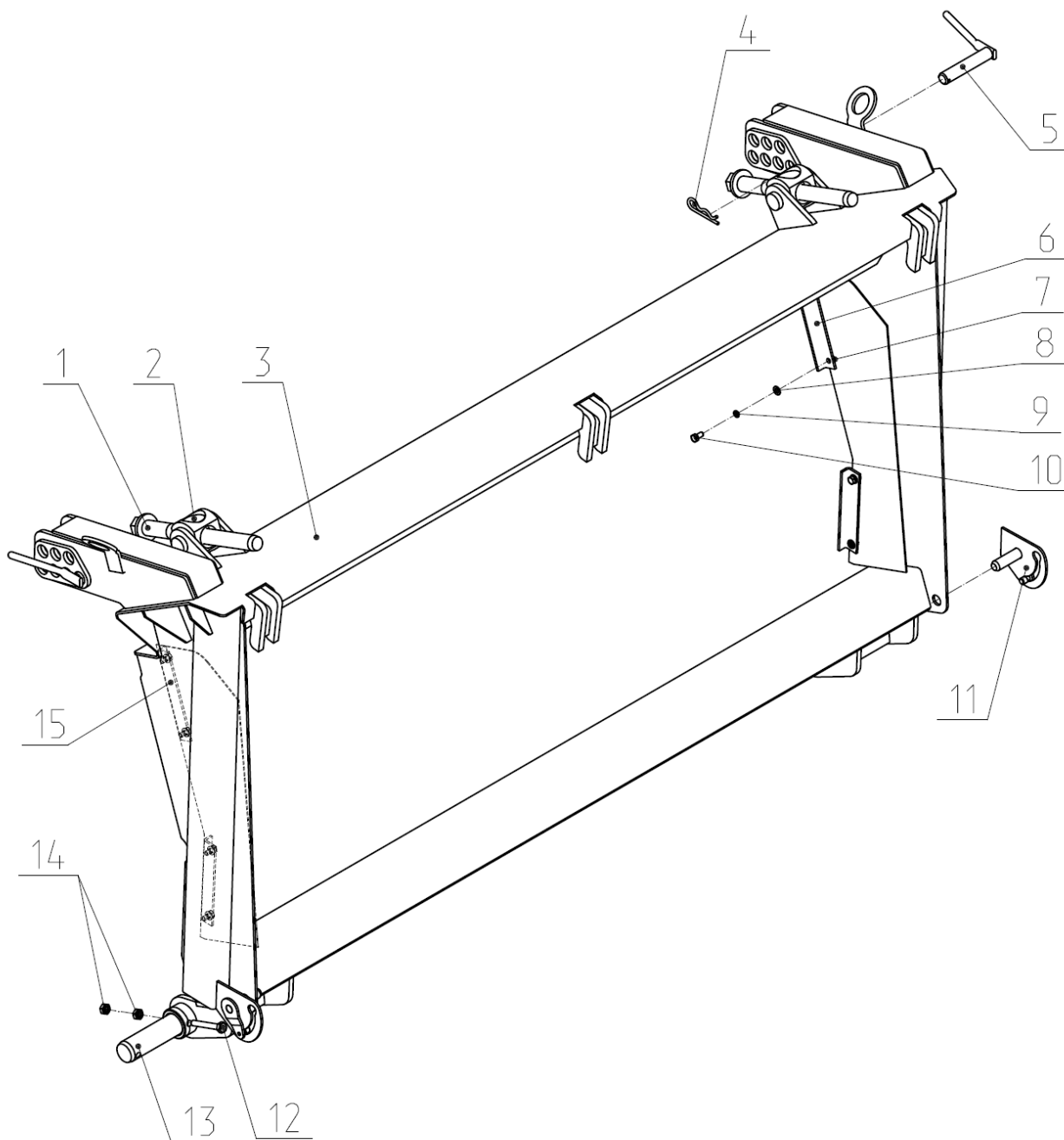
Рис. 16 ЖНПС 09.000 Адаптер.
