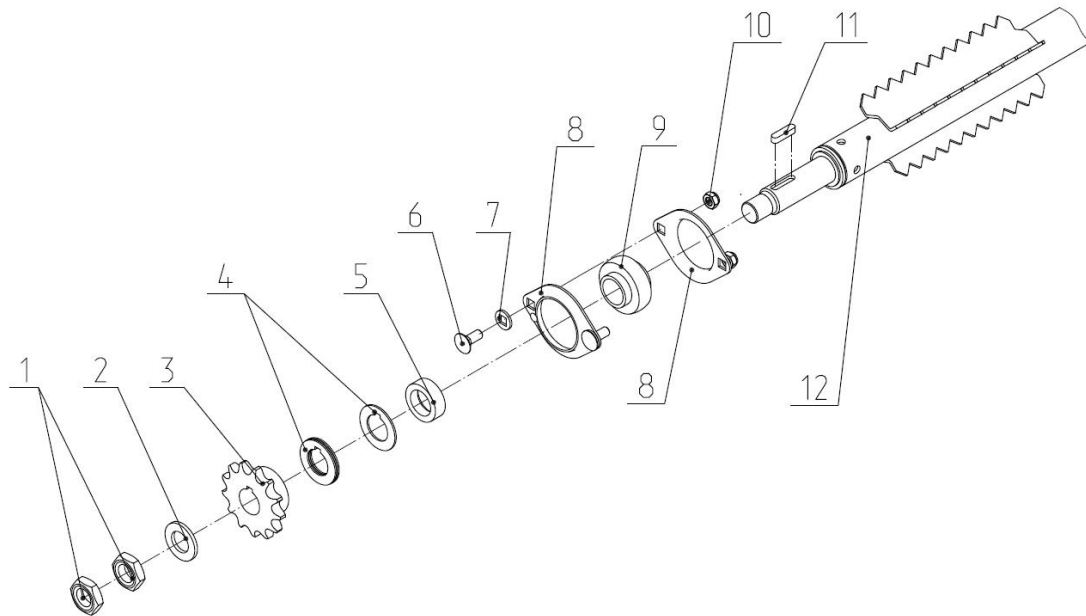
Рис. 5.1 Вал протягивающий на боковине справа.
