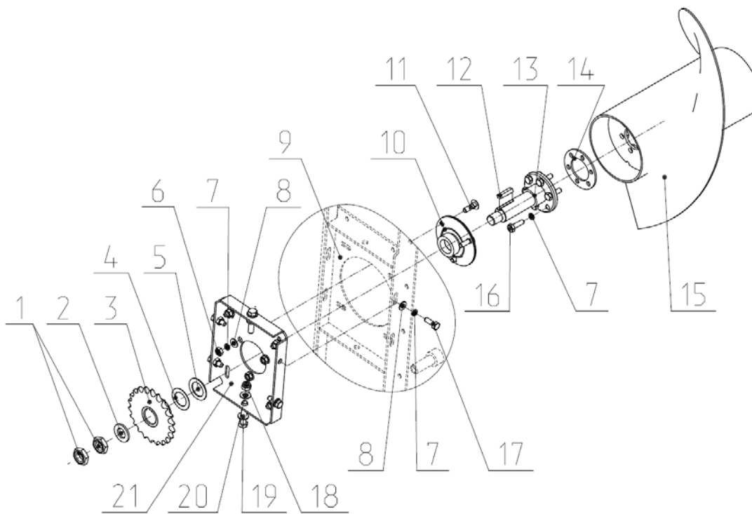
Рис.13.1 ЖНС 04.000 Шнек в сборе.
