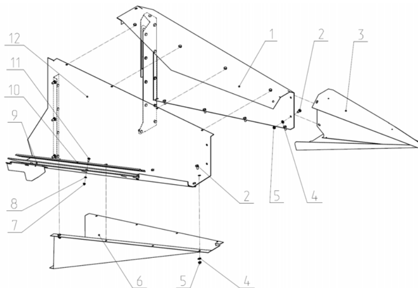
Рис. 4.1 ЖНПС 02.070 Пиллета.
