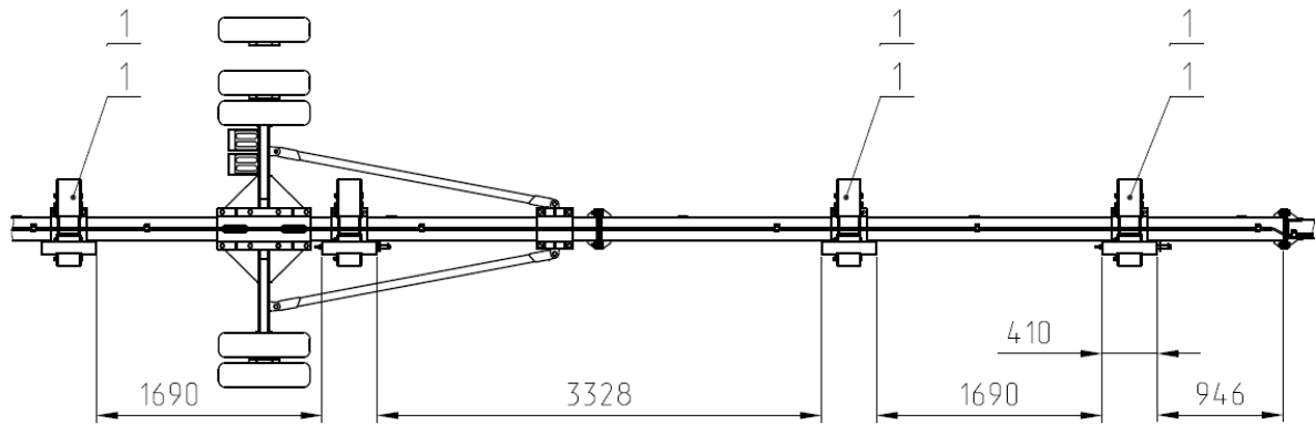
См. РЭ ТТ-3000 Рис. 17 РЭ ТТ-3000 Вид сверху приспособления. 1-Опора.
