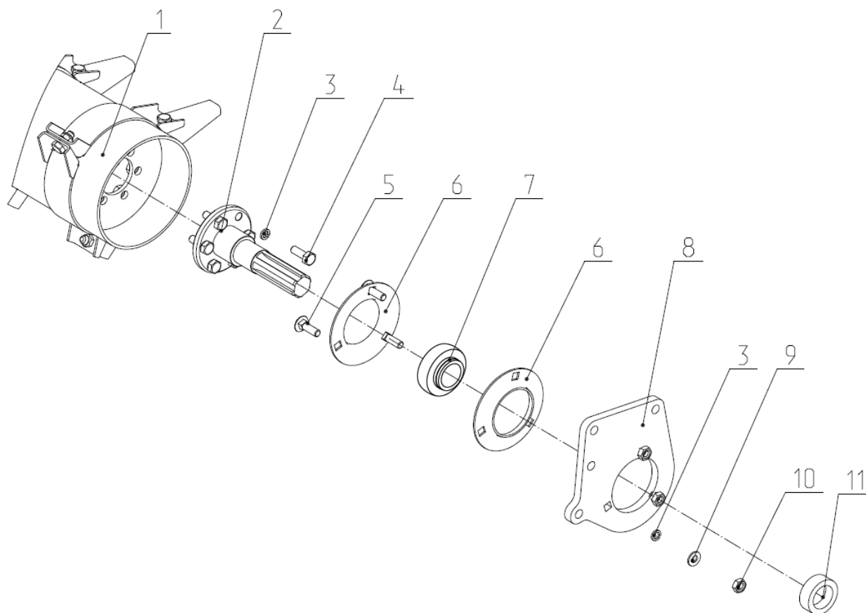
Рис.10.2 ЖНПС 03.020 Мотовило.
