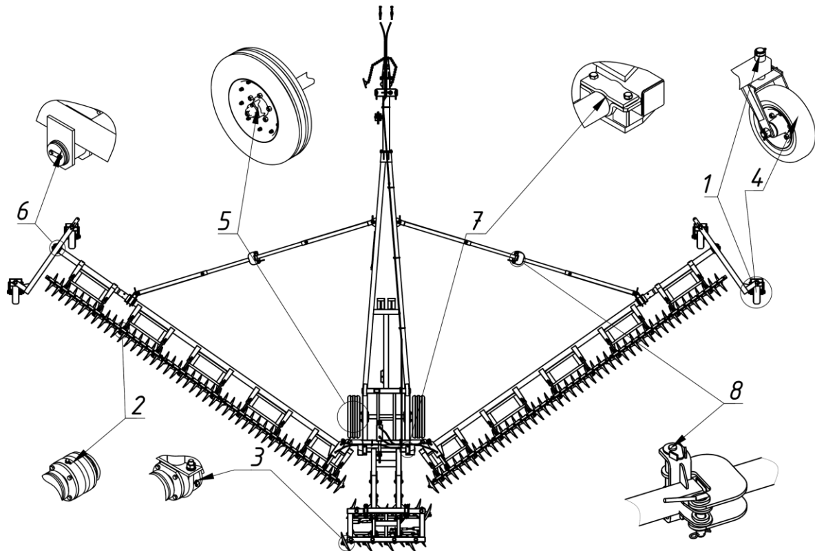
Рис. 23 Схема смазки
